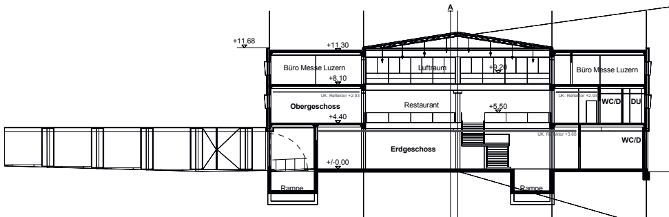
Halle 3 / Querschnitt
