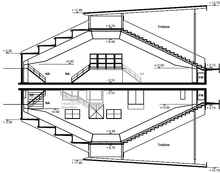
Halle 4 / Querschnitt West
