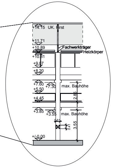
Detailsicht Schemaschnitt A-A (vergrößert)
